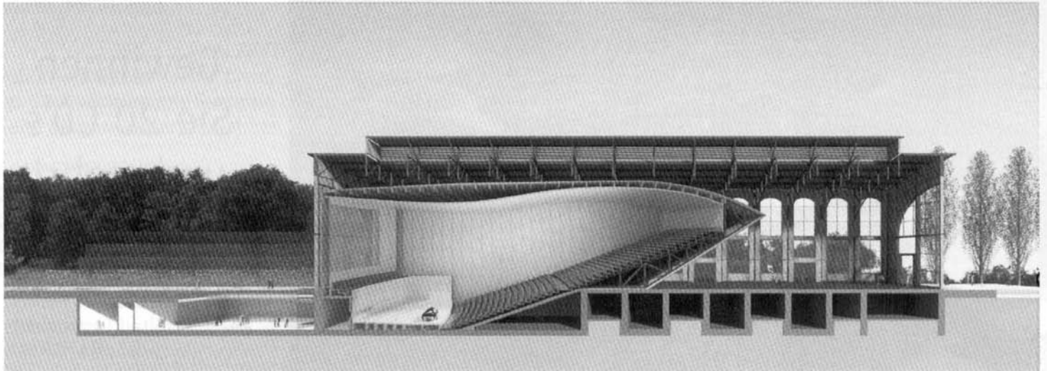
Querschnitt der neuen Philharmonie in Saarbrücken
